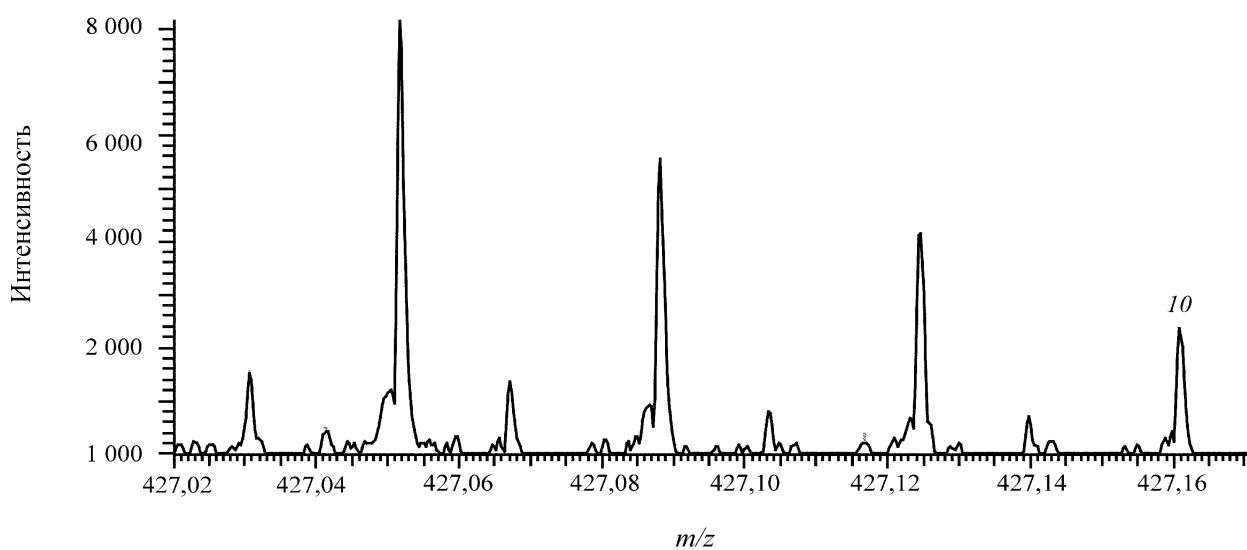
Рис. 2. Фрагмент масс-спектра образца ГВ природных вод 1R101N в диапазоне масс 427,02000–427,17000 а.е.м. Растворитель – ацетонитрил, концентрация 120 мг/л, потенциал ЭР 3,2 кВ
